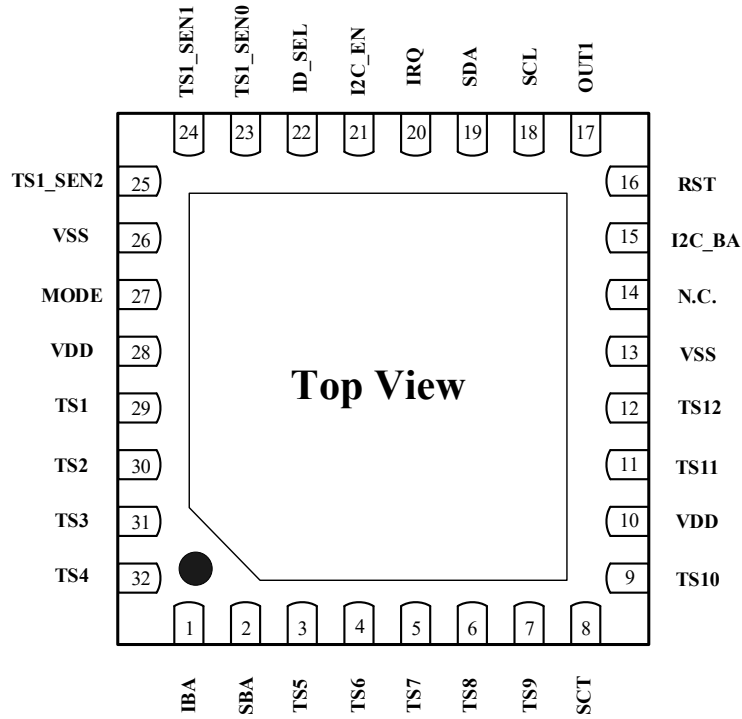
图 5.1 Si12T 管脚示意图（5x5 mm QFN32）
