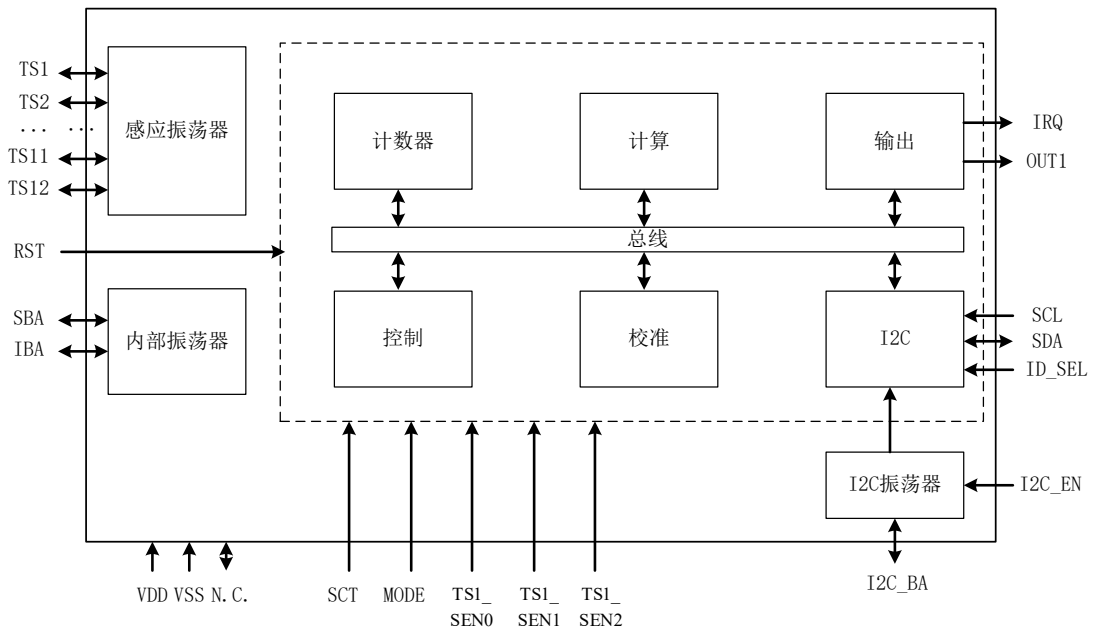
图 3.1 Si12T 简化框图
