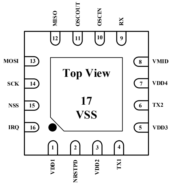
图 1-2 引脚配置图 (QFN16 3×3)
